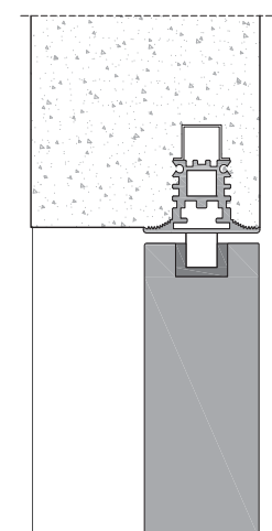
muratura ■ brickwall
