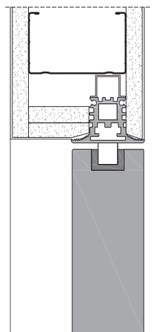
cartongesso ■ drywall
