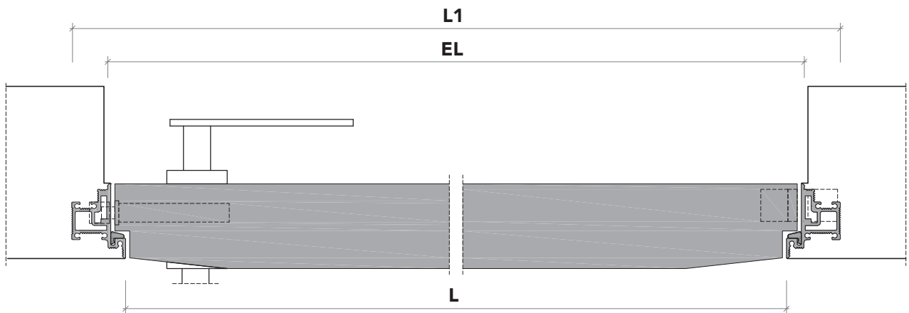
sezione orizzontale ▪ horizontal section
