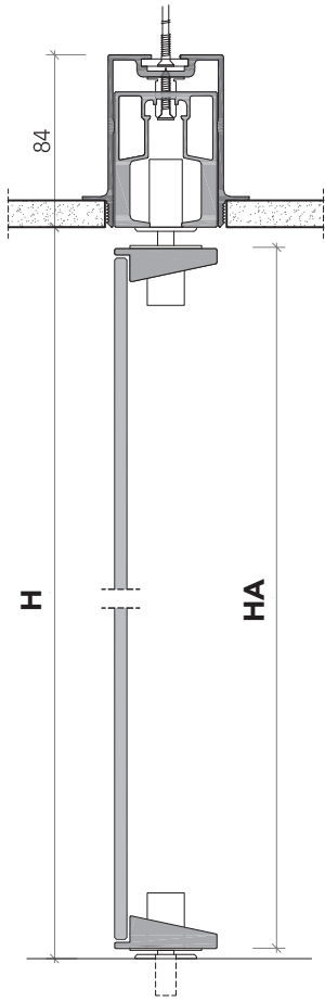
binario ad incasso ■ concealed rail
