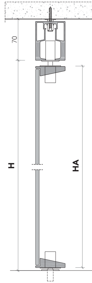
binario esterno ■ external rail
