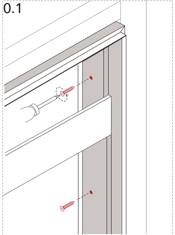
0.1 Fissare il falso telaio ai montanti con le viti. Fix the subframe to drywall beams with screws.
