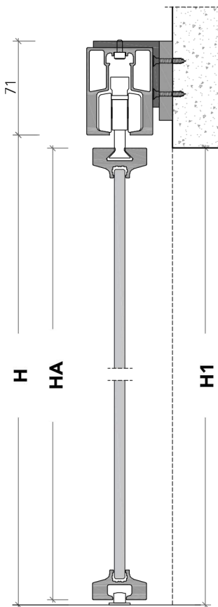
binario a parete ■ wall rail
