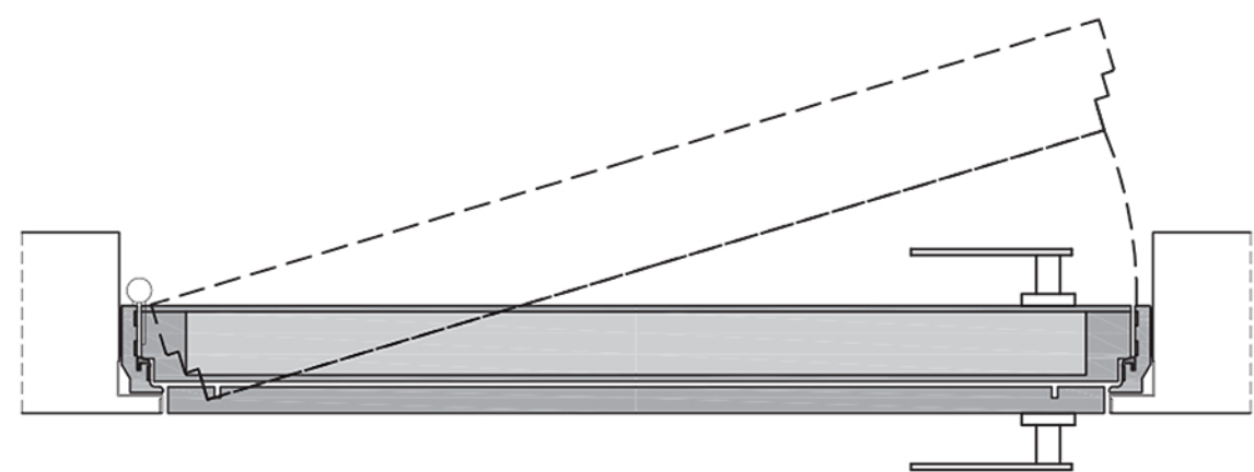
spingere sinistra ■ push left
