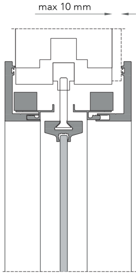
parete con rivestimento - cladding wall version
