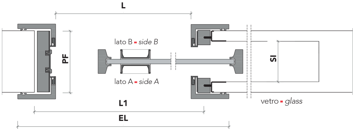
sezione orizzontale - horizontal section
