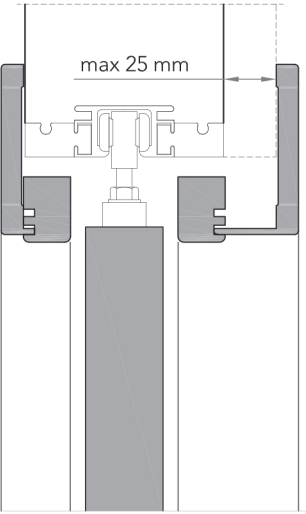
parete con rivestimento ■ cladding wall version
